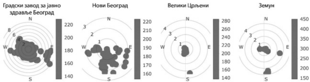
Слика 33: Зависност прекорачења сатних граничних вредности NO_2 [ \mu\text{g}/\text{m}^3 ] од компоненти ветра за период од 2017. до 2019. године
