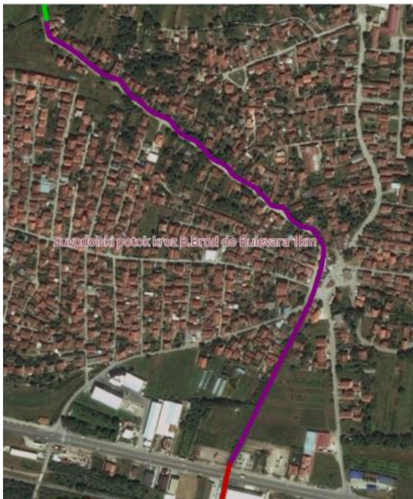
Суводолски поток кроз Брзи Брод до Булеvara Медијана L=1,0 km
