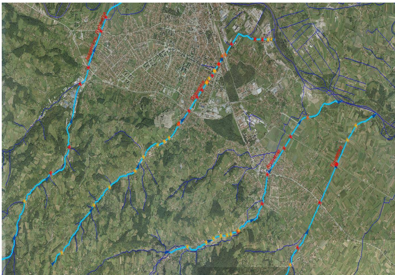
Слика 8. Критичне деонице за водотоке II реда где је смањен протицај
