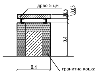
Детаљ клупе
