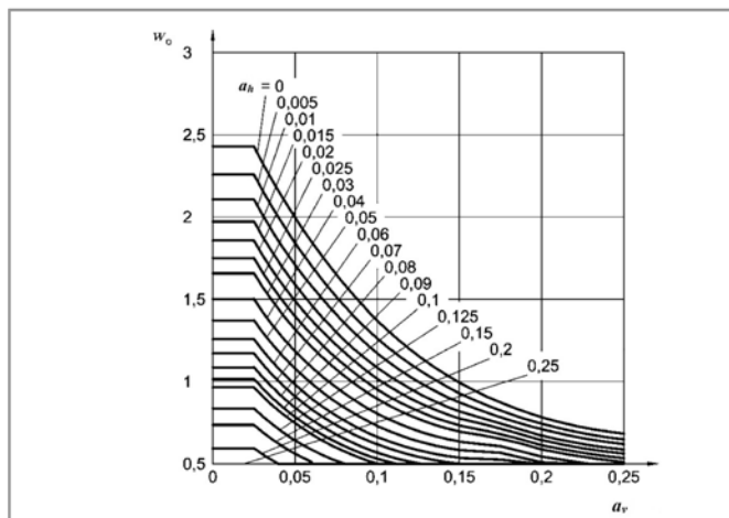
Слика 1. Фактор w_0 у зависности од a_v и a_h
